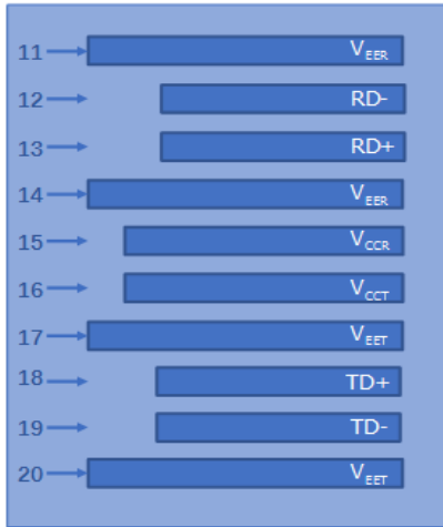
顶部视图
