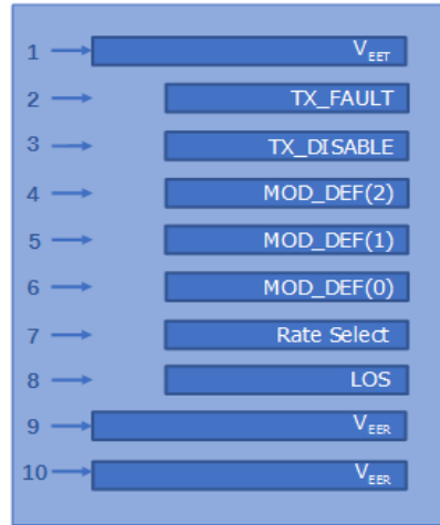
底部视图
